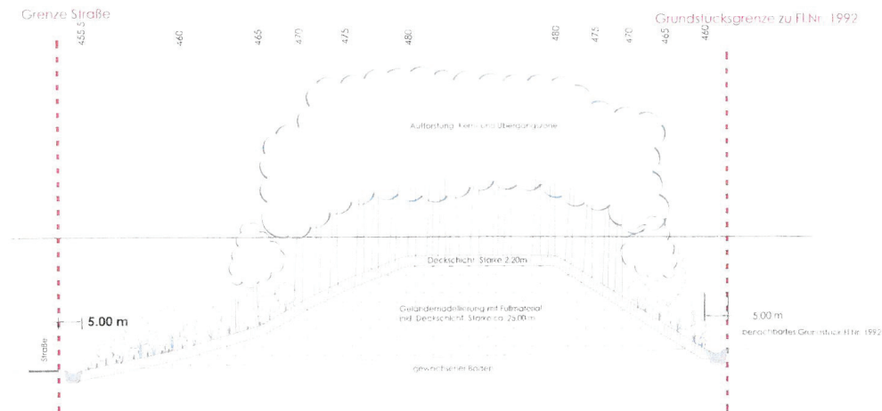
Schnitt C - C' Rekultivierung M 1 : 500
