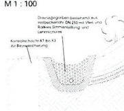
Detail 2 Drainagegraben am Fuß der Geländemodellierung Nord-West-Süd M 1 : 100
